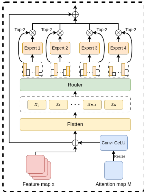
Fig. 3. MGS-MoE module
