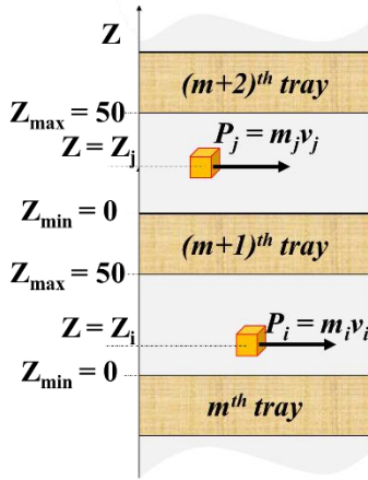
Fig. 3. Air spacing
