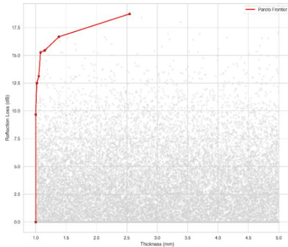
Fig. 3. Pareto frontier
