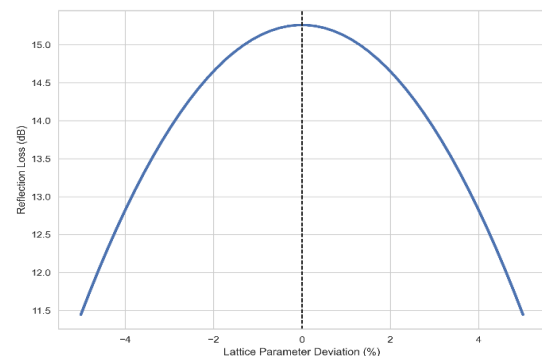
Fig. 7. Robustness
