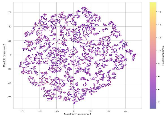
Fig. 8. Global manifold
