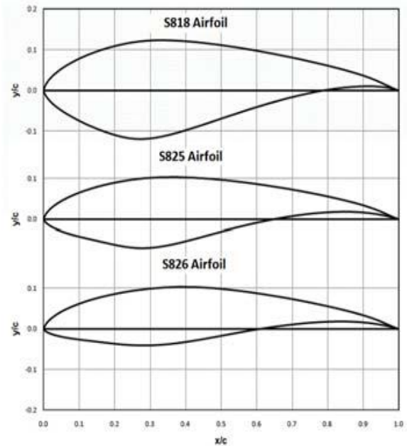
a. Airfoil
